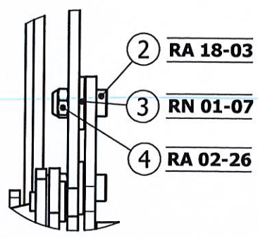
DETAIL A 1 : 2
